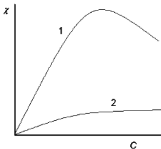
Рис. 1. Зависимость удельной электропроводности \chi от концентрации для растворов сильного (1) и слабого (2) электролита
