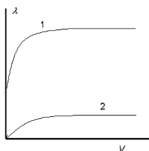
Рис. 2. Зависимость молярной электрической проводимости \lambda от разбавления для растворов сильного (1) и слабого (2) электролита
